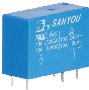
Ρελέ 12V DC 10A
